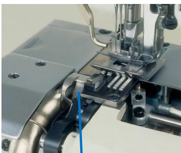
FT0C, Kantenbeschneider links der Nadeln
